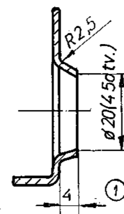
Presek A-A M1:1
